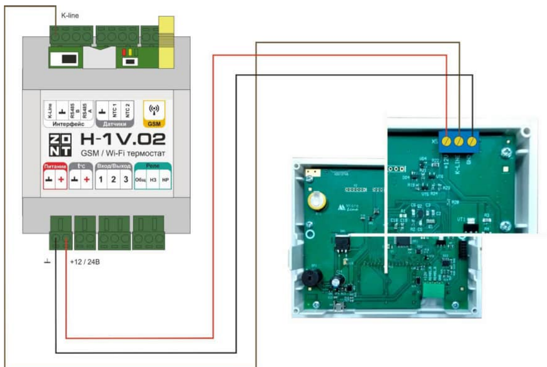
Интерфейс K-Line
